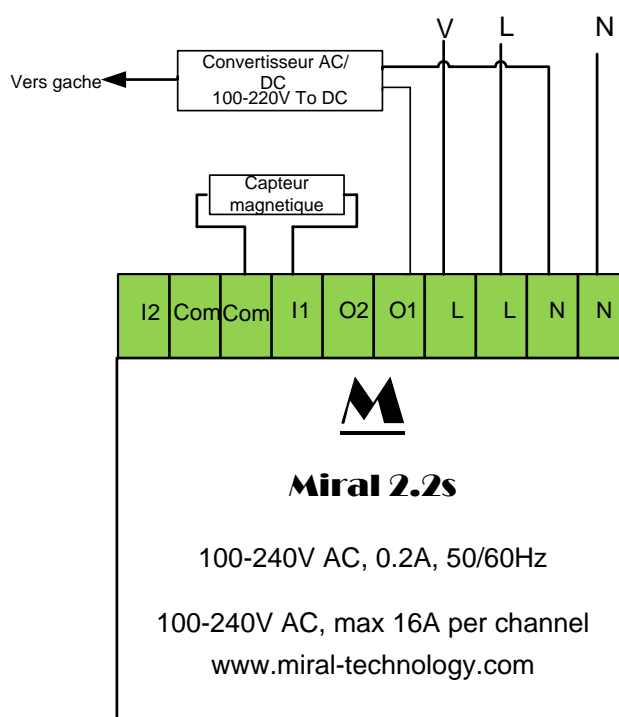
Figure 4: Branchement pour le control d'une gâche de porte
