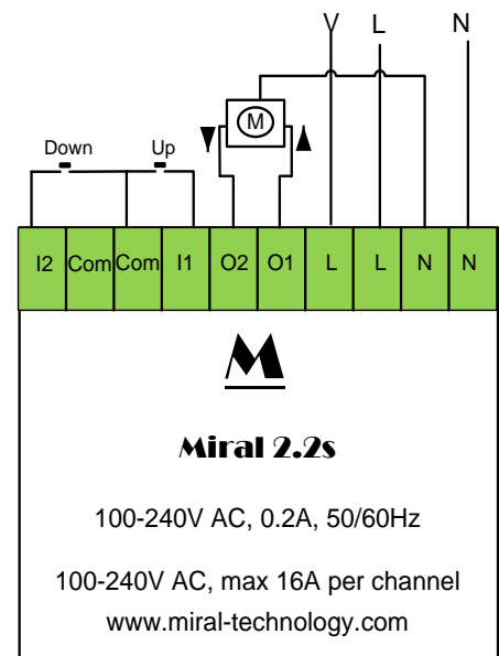
Figure 2: Montage pour le control d'un moteur
