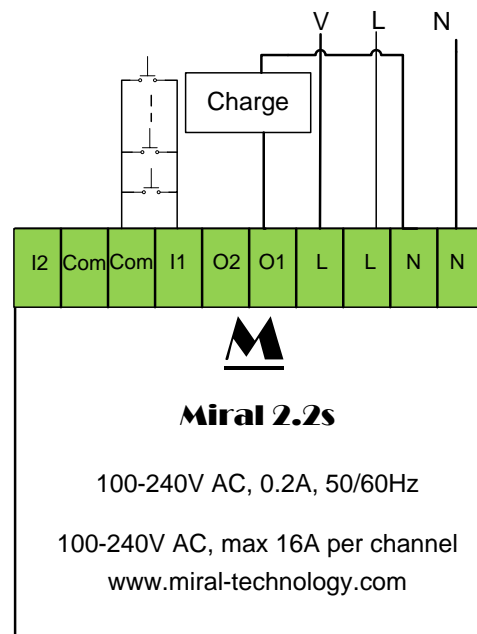
Figure 5: Branchement pour le control d'une charge en mode télérupteur
